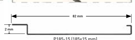
P185-15 (185x15 mm)
