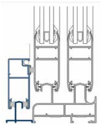
GUIA SIMPLE (PERMET MULTICARRIL EN PARAL·LEL)
